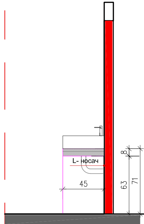
ПРЕСЕК 1-1
