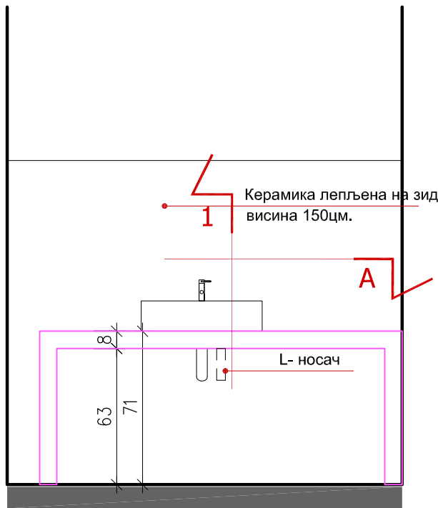
ИЗГЛЕД Ц-Ц
